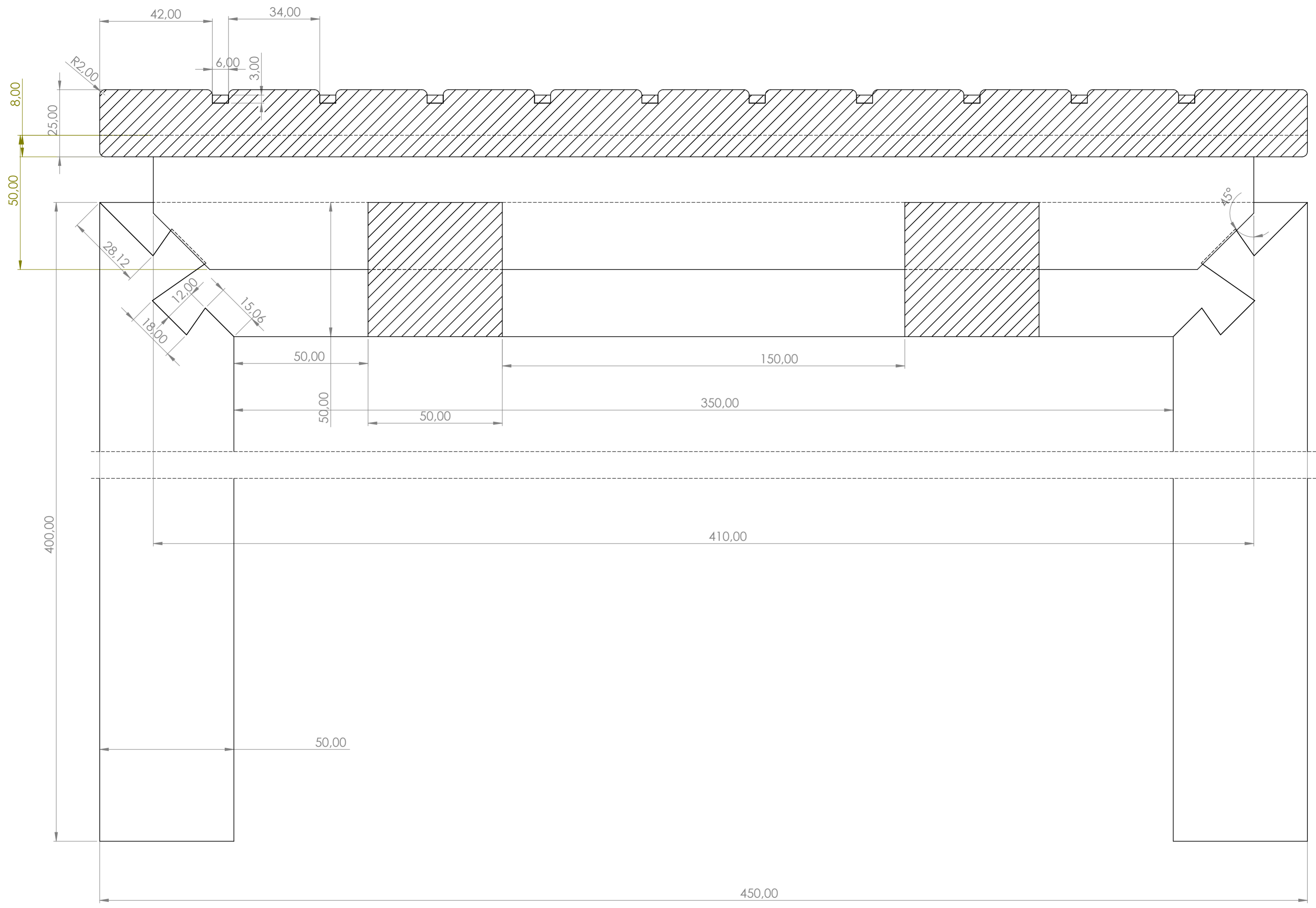
SECTION A-A SCALE 1 : 1
